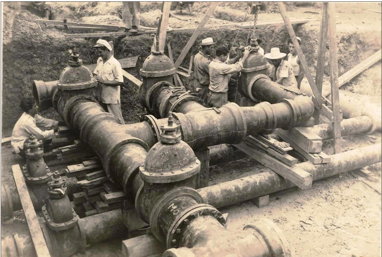
Tanques y red de distribución de agua a la ciudad de P. del Río, construidos en 1906. Foto de archivo.
